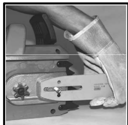
(1)-Линейка; (2)- Зазор; (3)- Нет зазора; (4)-Отклонение цепи.
